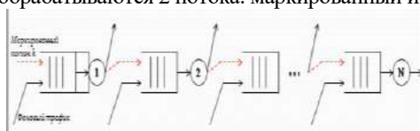
Рисунок 1 - Сеть с тандемной очередью
