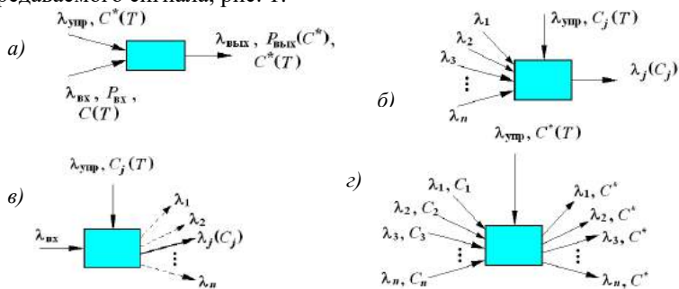
Рисунок 1 – Схемы функционального преобразования «форма сигнала \leftrightarrow функция чирпа»: а – приобретение заданного чирпа C^* ; б – выбор длины волны \lambda_j из заданного набора, соответствующей j -ой функции чирпирования C_j ; в – преобразование \lambda_{вх}/\lambda_j в зависимости от C_j ; з – функция «копирования чирпа», передаваемого всем длинам волн от управляющего сигнала (на входе присутствуют сигналы с произвольным чирпированием)
