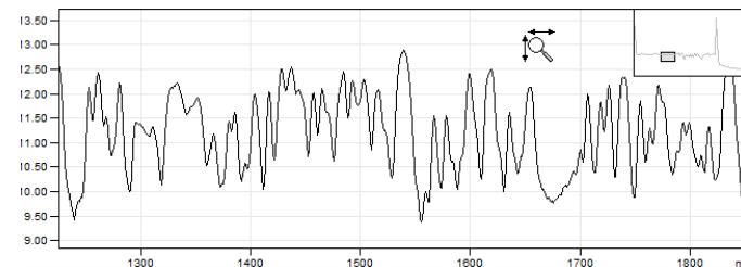
Рисунок 1 - Пример поляризационной характеристики обратного рассеяния
