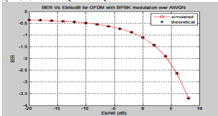
Рисунок 2 - Отношение между SNR и BER для OFDM с BPSK в AWGN
