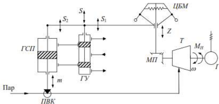
Турбогенератордың бұрыштық жылдамдығын тұрақтандыру жүйесінің функционалдык сұлбасы
