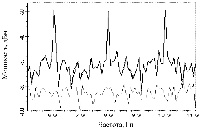
Рисунок 2 - Отклик трех ВБР с различным разносом фазовых сдвигов. Построенные на базе указанных решеток сенсорные сети, аналогичные рассмотренным в [1,2] не требуют использования спектральных или интерферометрических интеррогаторов.
