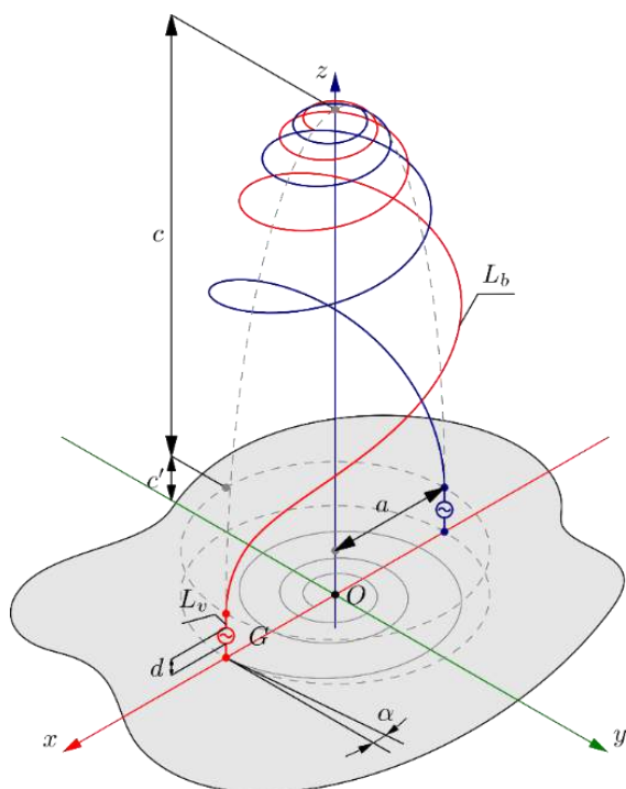
Рисунок 1 - Геометрия двухпроводного спирального эллиптического излучателя
